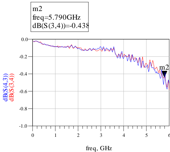
- S-parameter -
