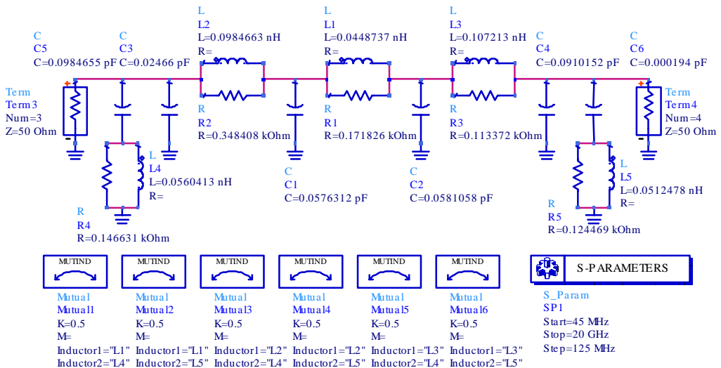
- S-parameter -
