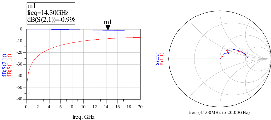
- S-parameter -
